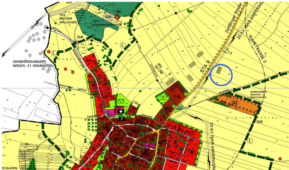
Ausschnitt des rechtsgültigen Flächennutzungsplans (Stand 14.12.2004) mit Planungsgebiet (blaue Markierung)
